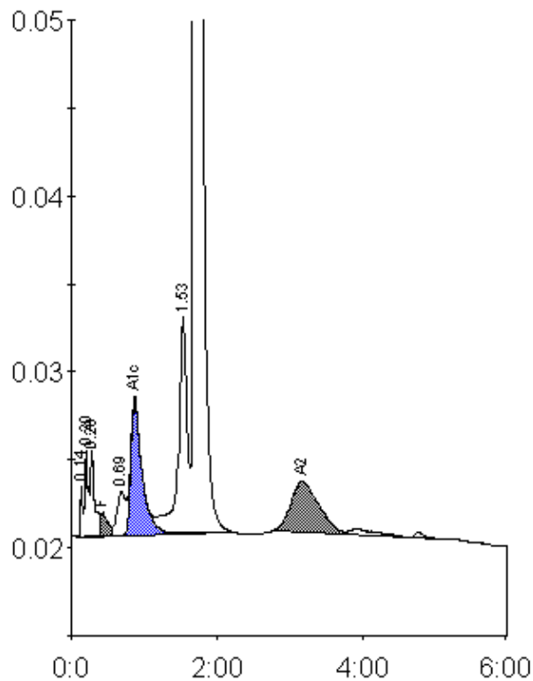
Peak table - ID: 10511961
